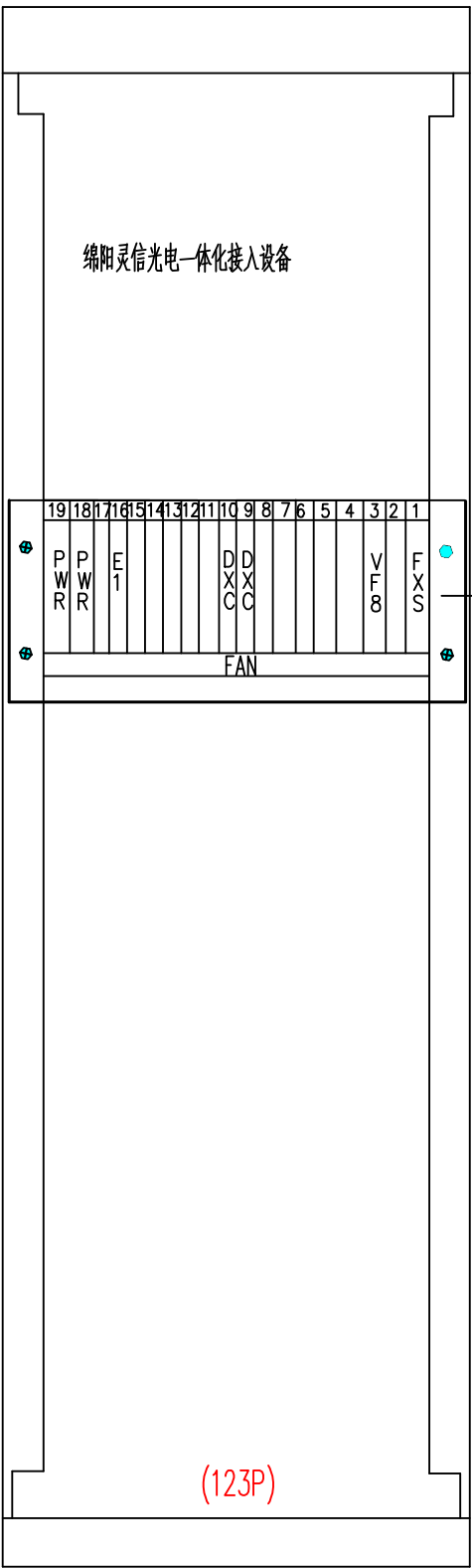
省网光电一体化设备机架图
